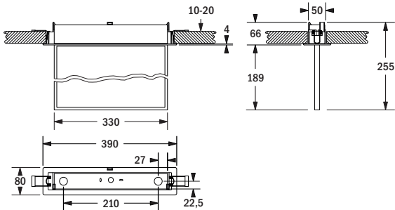
Deckeneinbau (Hohldecke)
