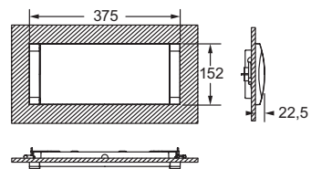
Wand-Ausnehmung 370 x 130
